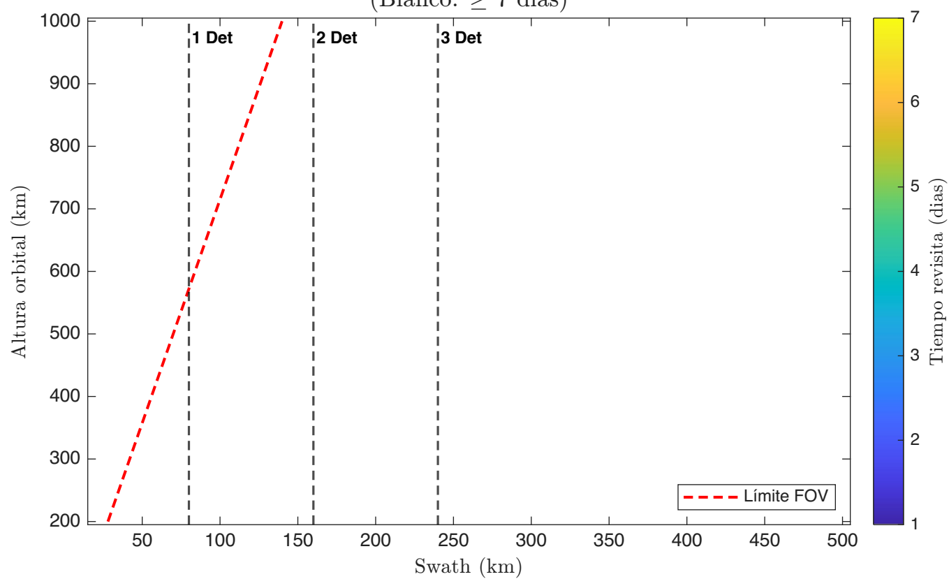
Tiempo Revisita - 1 Satelite(s); 1 Telescopio(s): TMA; Detector 3 (Blanco: \geq 7 dias)
